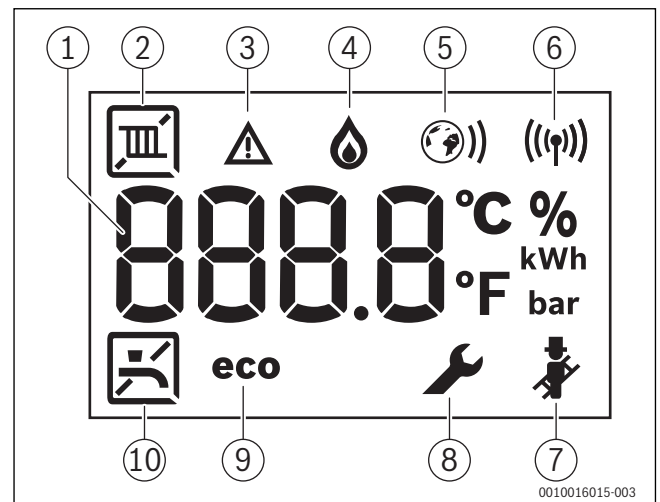
Rys. 2 Wskazania na wyświetlaczu
